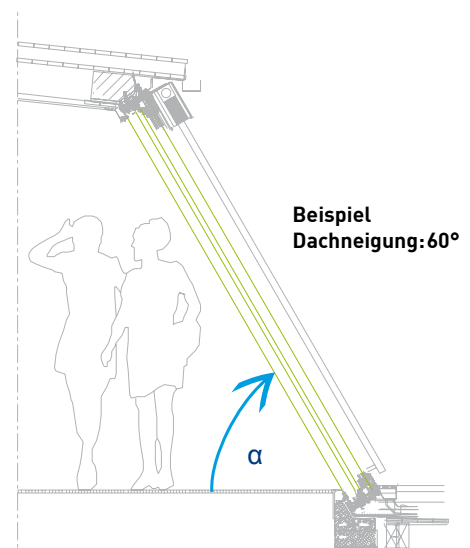
Vertikalschnitt
