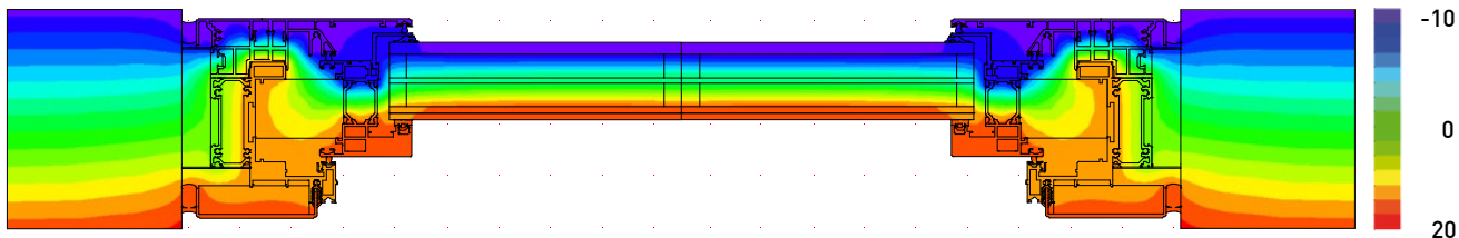
Isothermenverlauf
